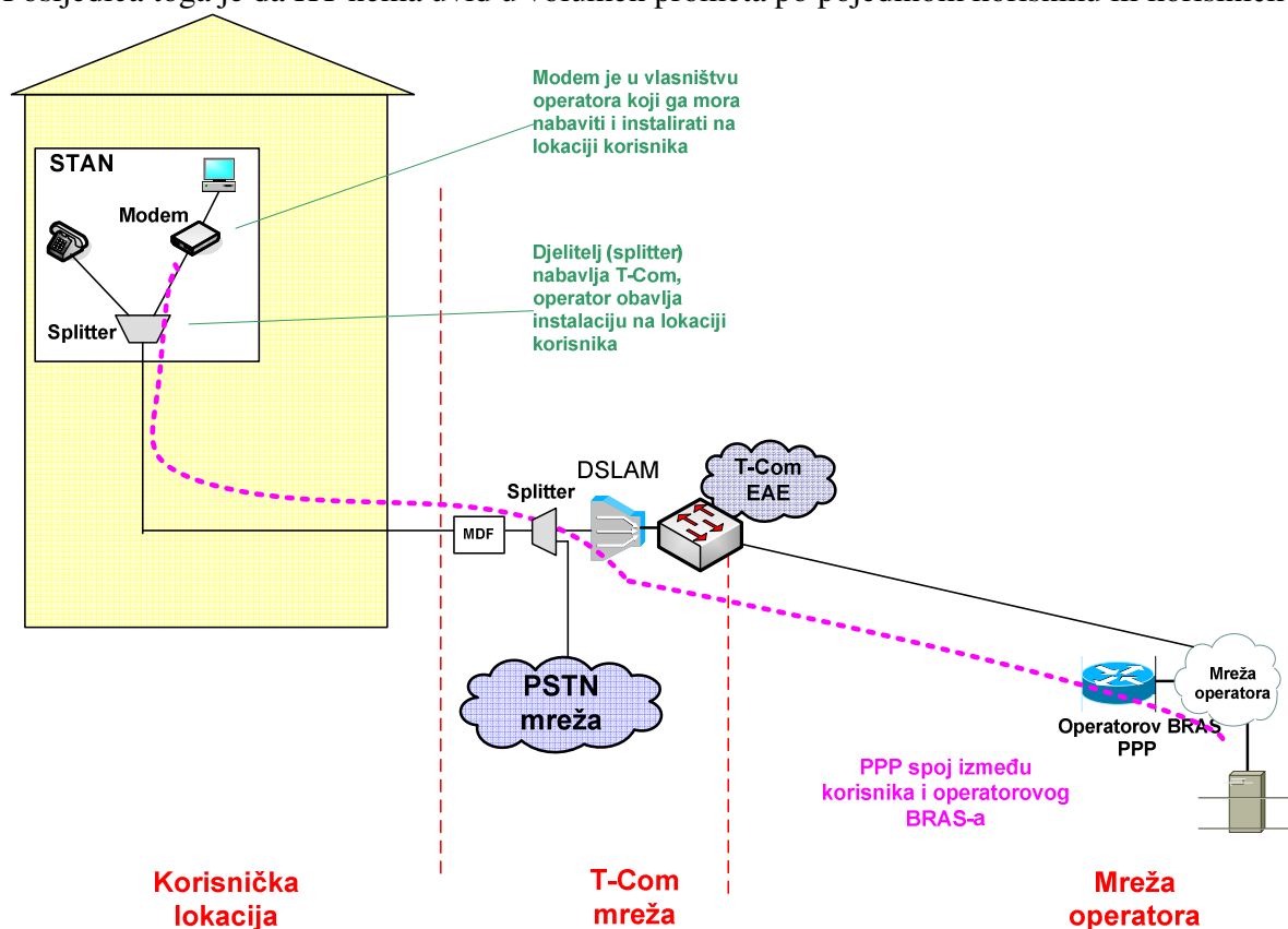
Slika 9. Način realizacije Veleprodajnog širokopojasnog pristupa za pružanje Internet usluge na DSLAM razini
